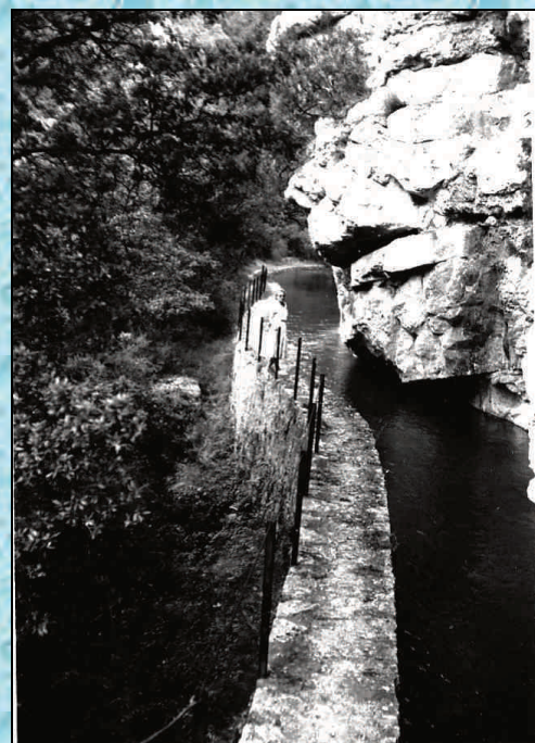
Le canal dans la gorge, contre la paroi sud en amont du tunnel de 260 m (dans le massif cote 466, face à la Côte de Vauclare, en 1959).
